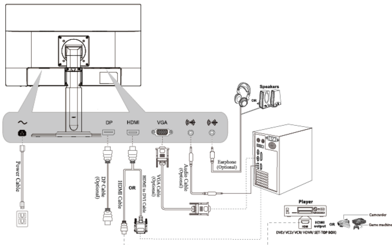
Figura 2. Branchement à un pc
